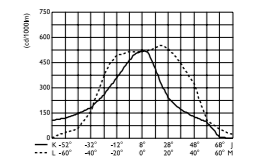
Sodium Haute Pression 100 W L.O.R. = 0,73 • 1 x 10700 lm
